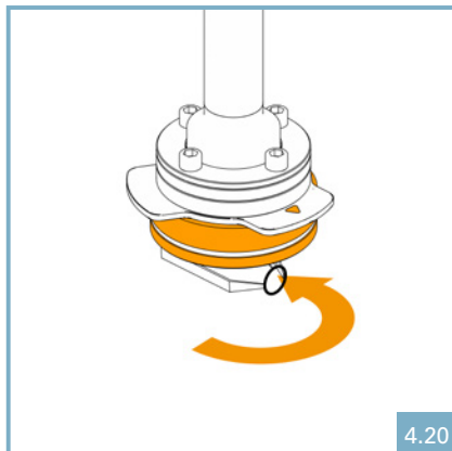
Molchfänger um 180° drehen.
