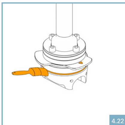
Dichtung am Bajonettverschluss mit Gleitmittel bestreichen.
